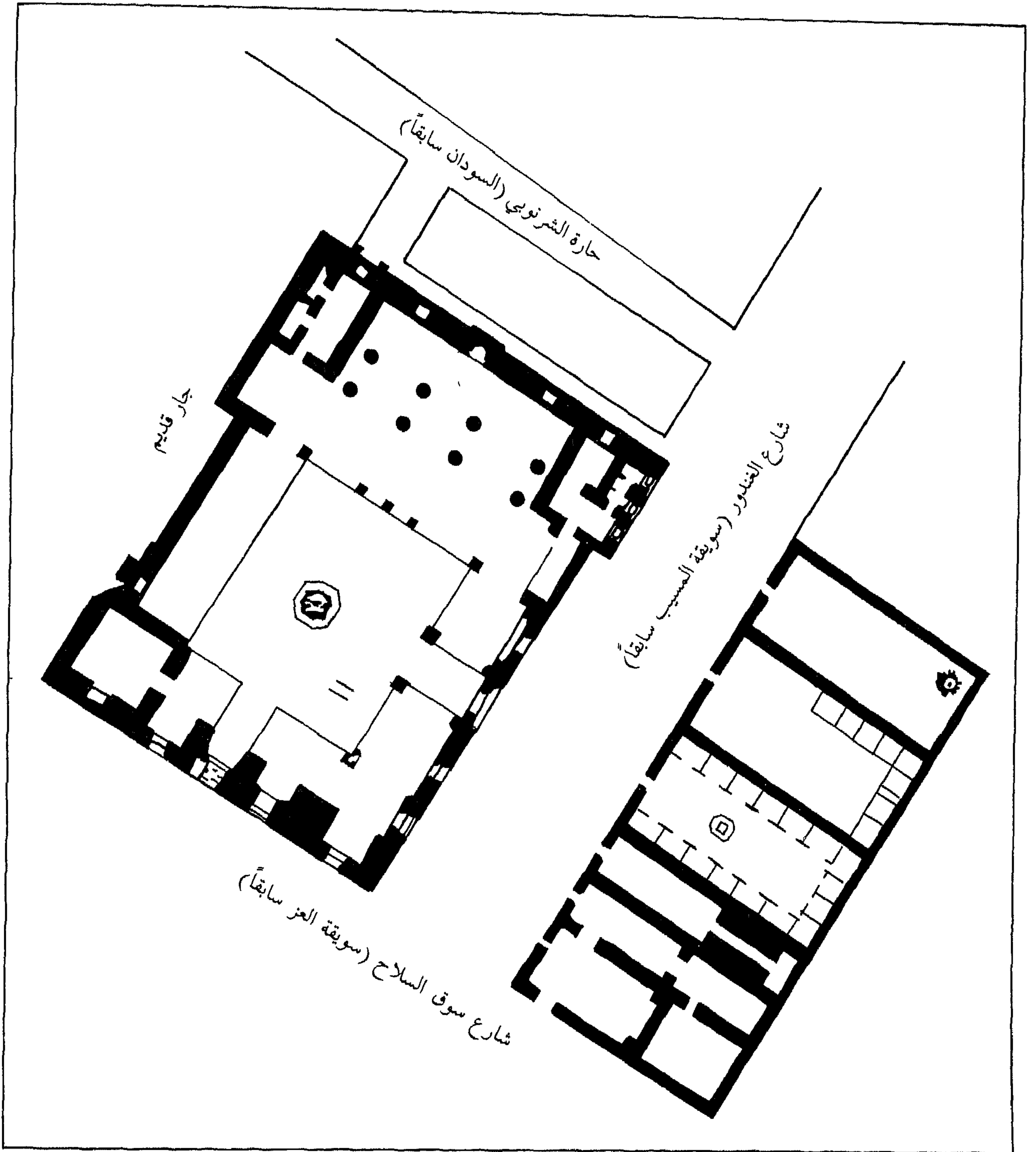
شكل (٧) تصور للمسقط الأفقي لمدرسة الأمير سودون من زادة وقت انشائها بما في ذلك الملحق الواقع على شارع الغندور استنباطاً من الحججة الشرعية للأمير والشواهد المعمارية الباقية.
